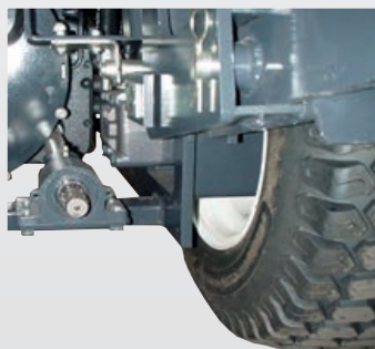
Trasm. anteriore completamente idraulica (Motore - Ruota)
