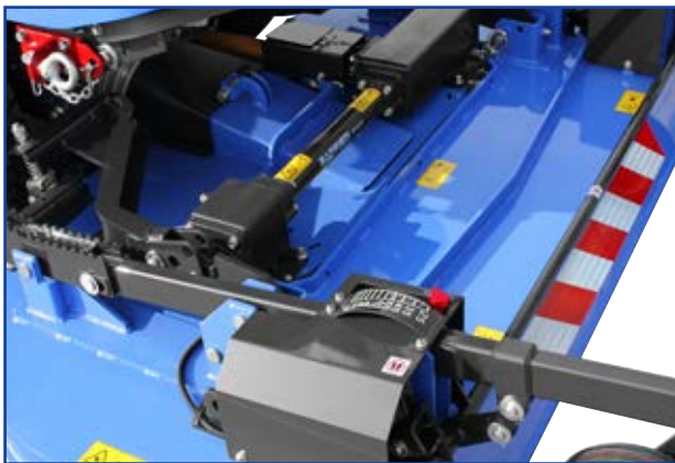
Regolazione "Elettro-idraulica del piatto dal posto guida
